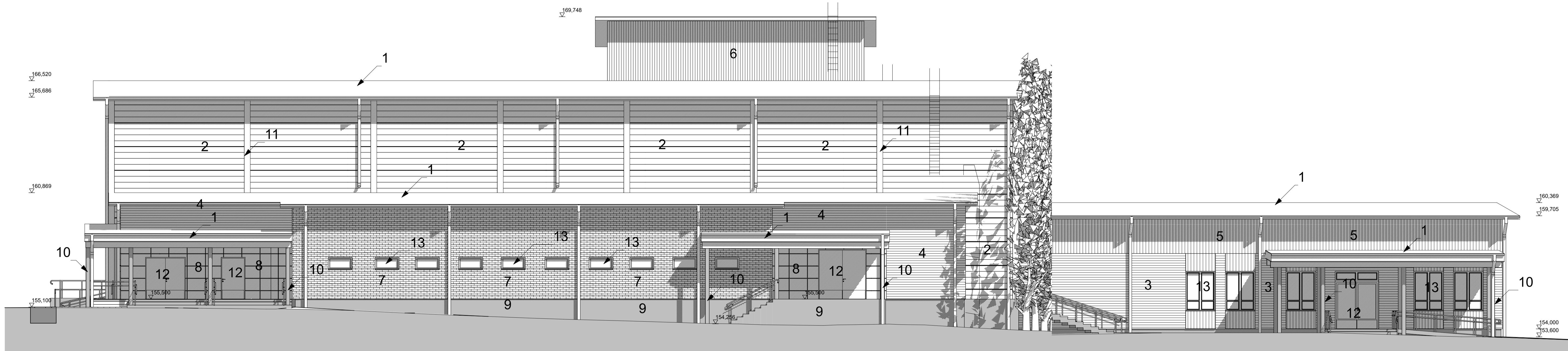
Julkisivu etelään
