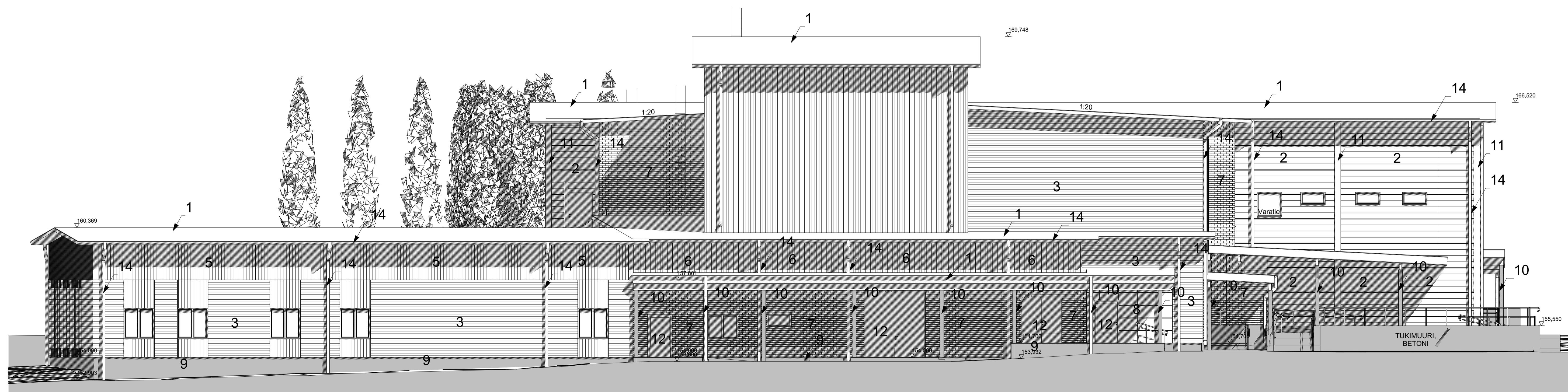
Julkisivu pohjoiseen
