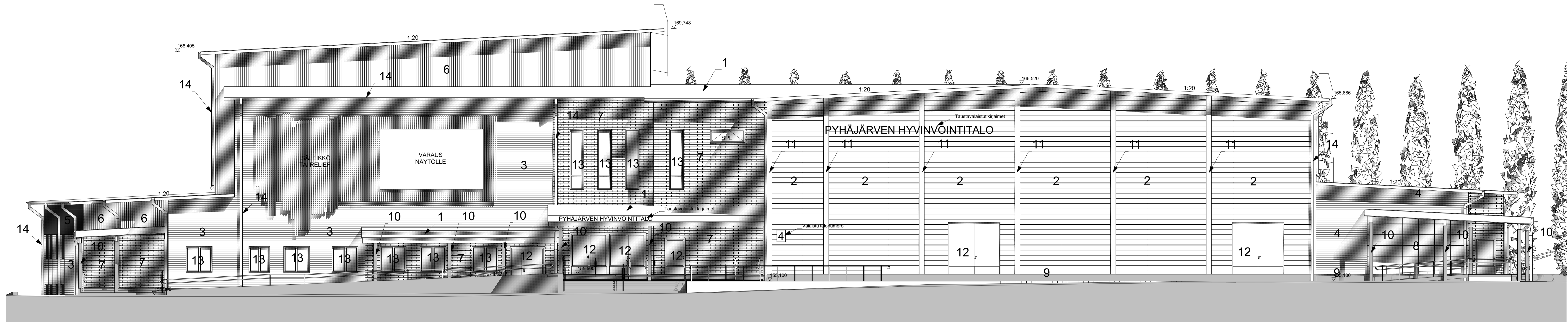
Julkisivu länteen
